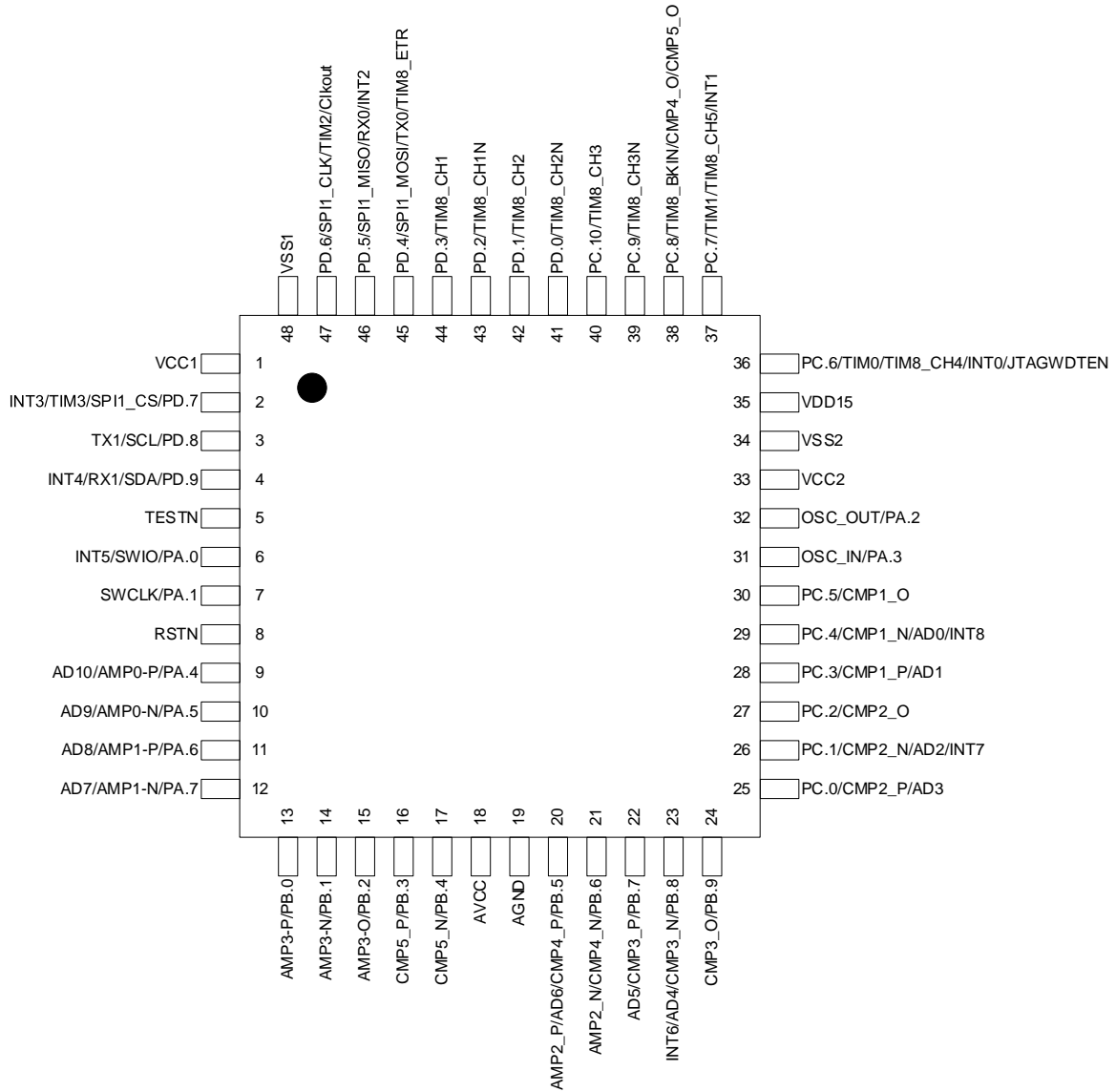
LQFP48
